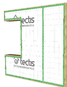
Tectis® VCL 5 Membraan afgeplakt met de Sitko Flex
